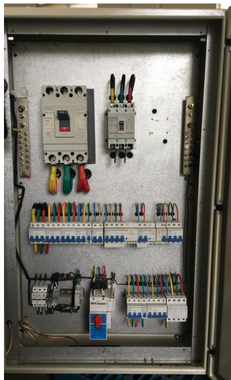
内部照片
