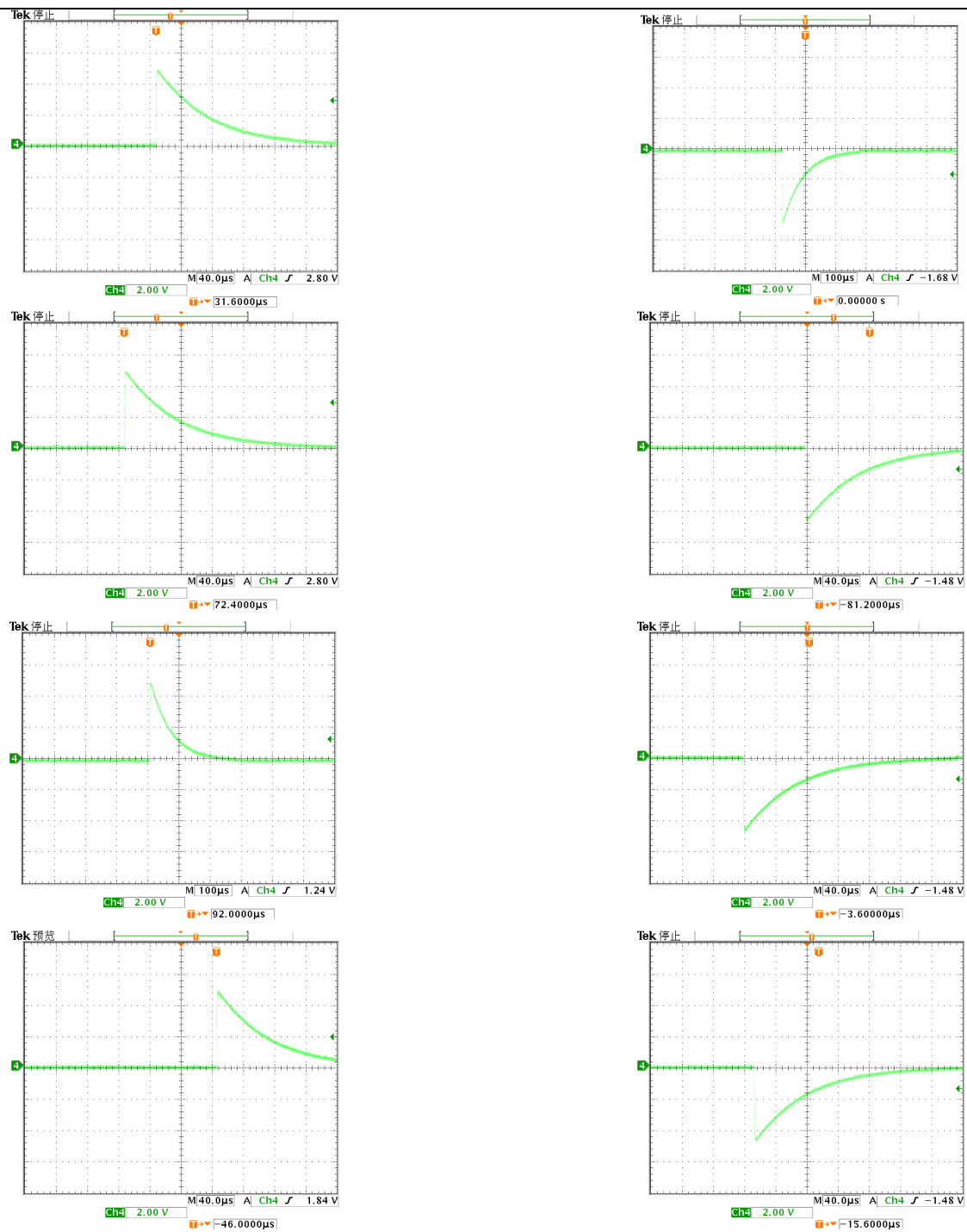
冲击耐受电压示波图
